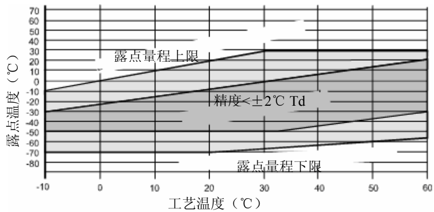
图32 DMP74B 精度
