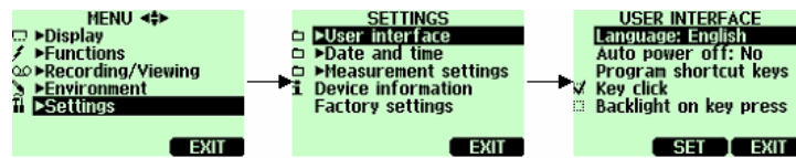
图14 用户界面
